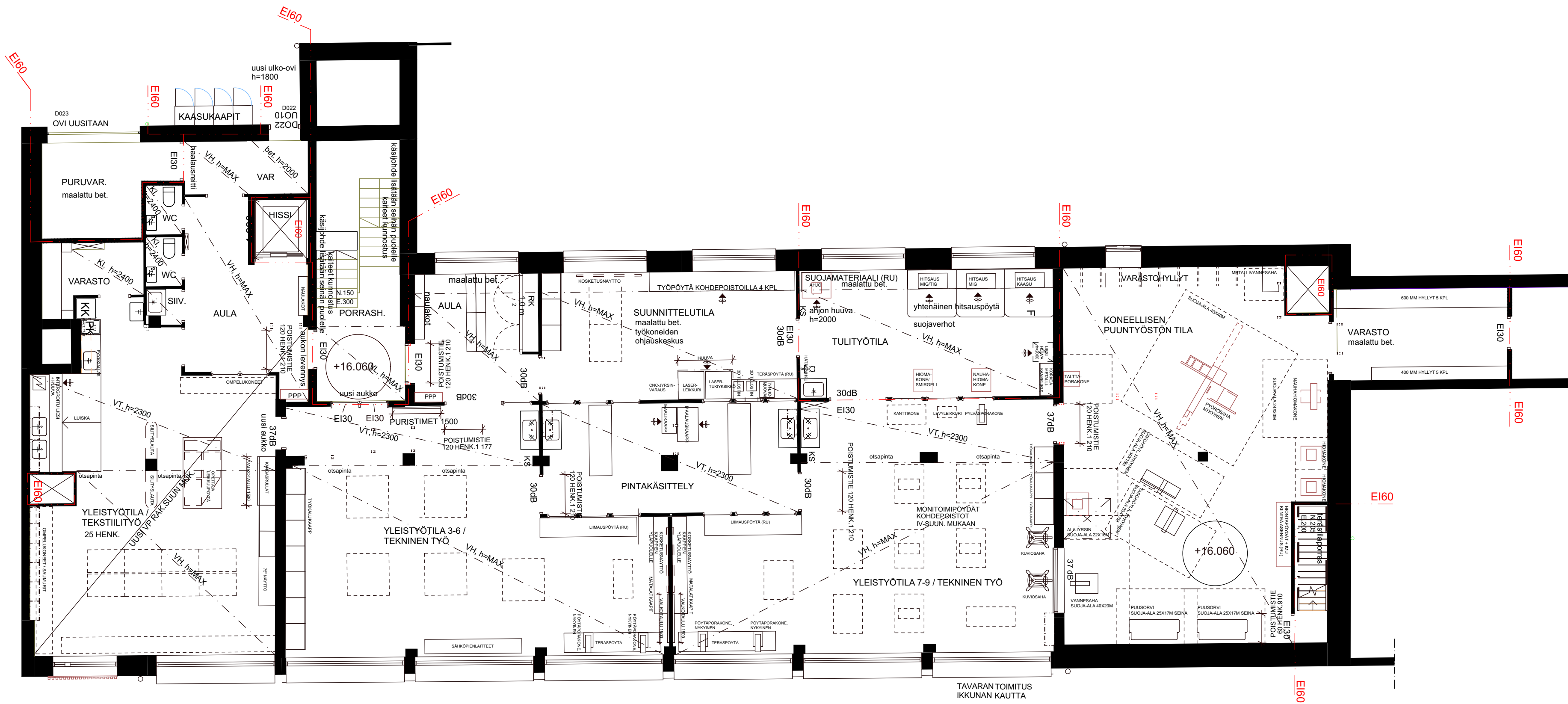
KÄSITYÖN OPPIMISYMPÄRISTÖ 1:100 (A2) PUOLALAN KOULU ARKKITEHTI: ARKKITEHTISUUNNITTELU MIKKO UOTILA KUVANKÄSITTELY: OPETUSHALLITUS 2023
